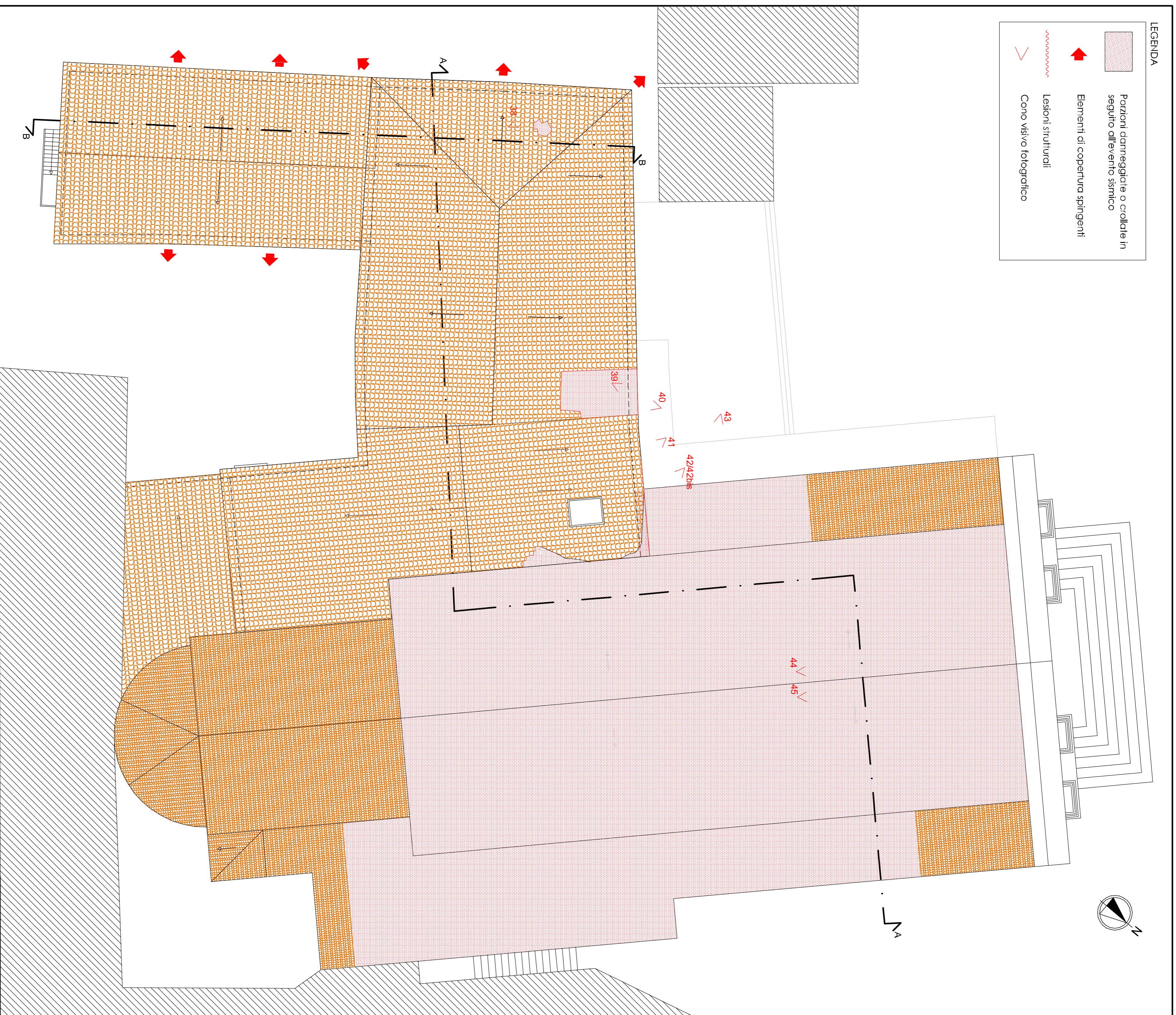
Pianta coperture
